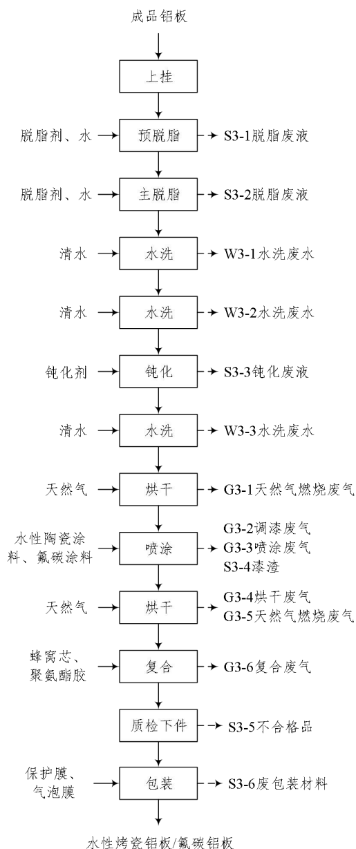
图 2-8 水性烤瓷铝板/氟碳铝板生产工艺流程图
