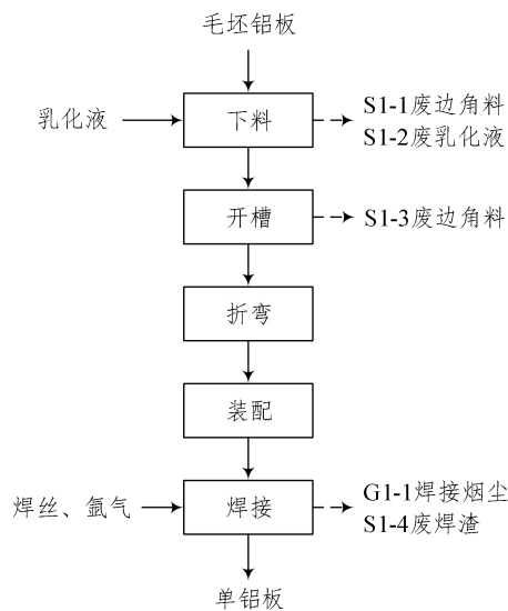
图 2-6 单铝板生产工艺流程图
