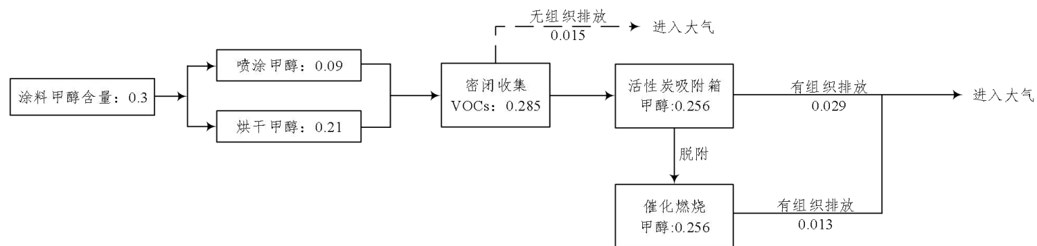
图 2-5 本项目甲醇平衡图 单位: t/a
