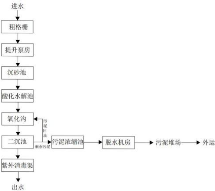
图 4-4 湟里污水处理厂处理工艺
