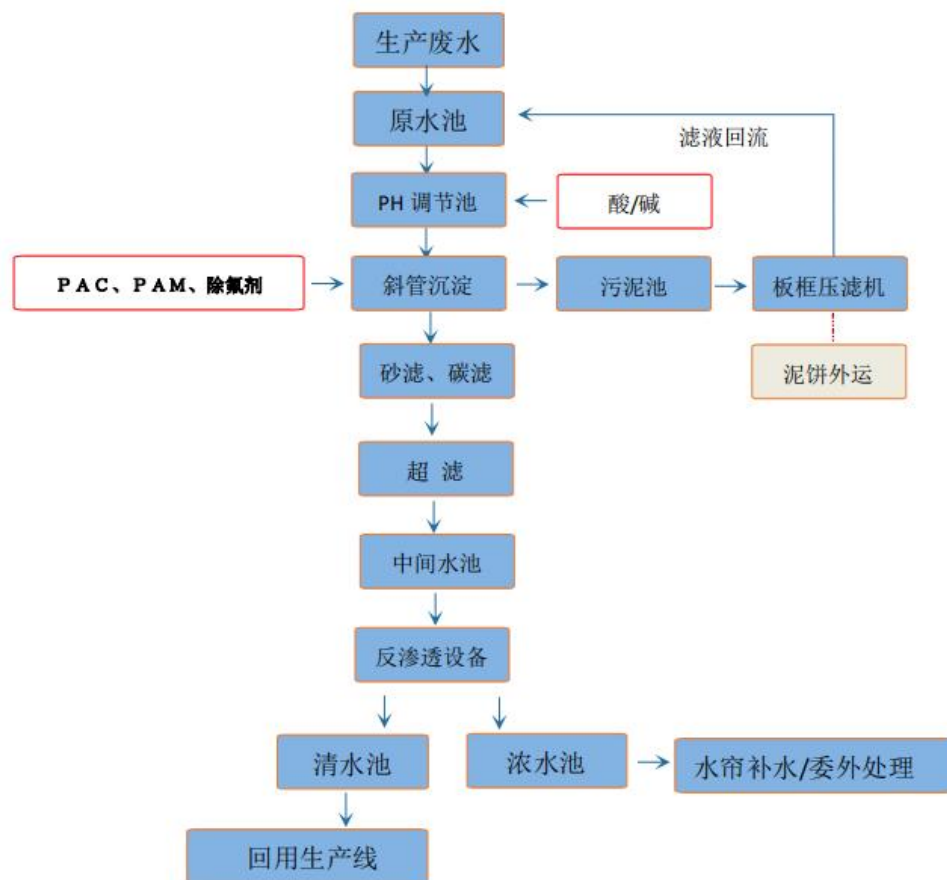
图 4-3 污水处理工艺流程示意图
