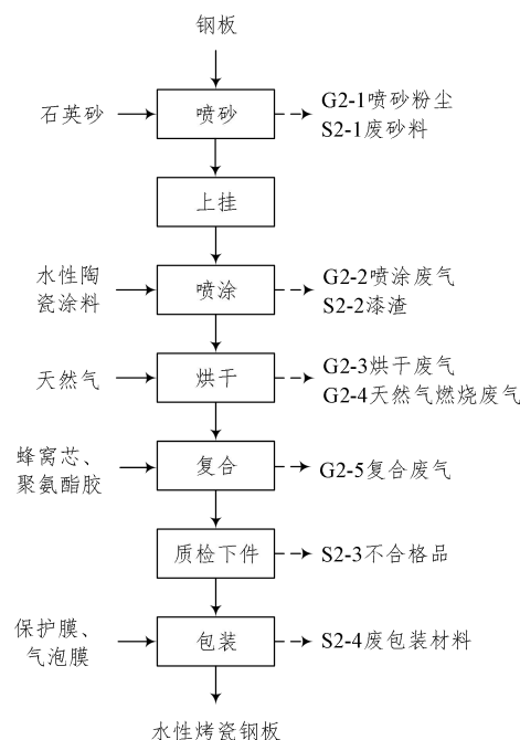
图 2-7 水性烤瓷钢板生产工艺流程图
