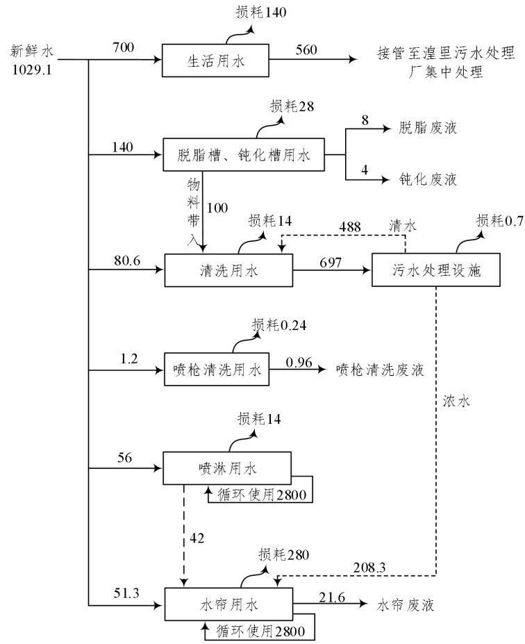
图 2-2 本项目水平衡图 单位 m³/a
