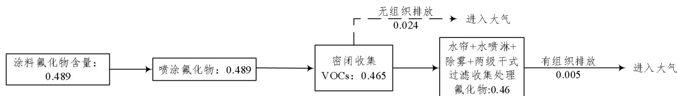
图 2-3 本项目氟化物平衡图 单位：t/a
