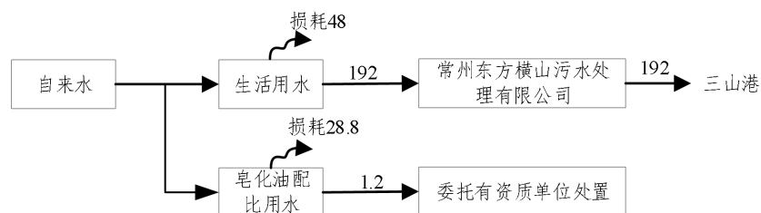
图 2-2 本次验收项目水平衡图 (单位 t/a)
