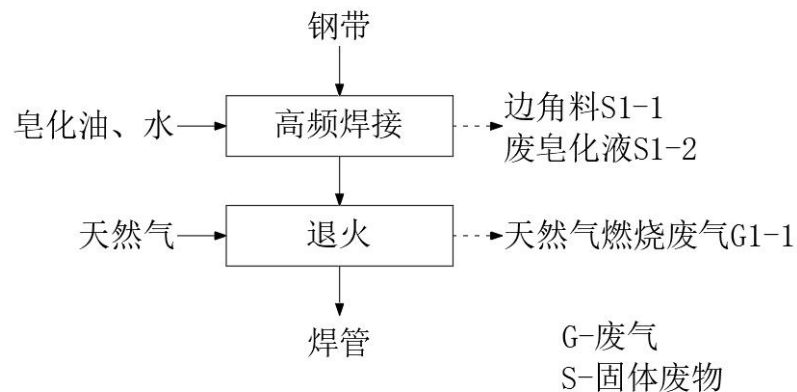
图 2-3 焊管生产线环评生产工艺流程图
