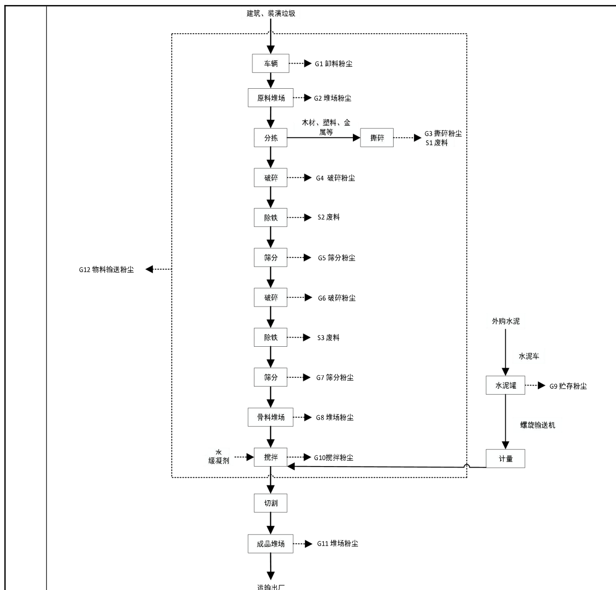
图 2-3 生产工艺流程图
