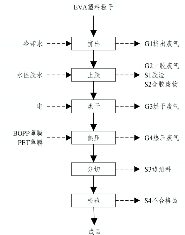
图2-3 工艺流程图
