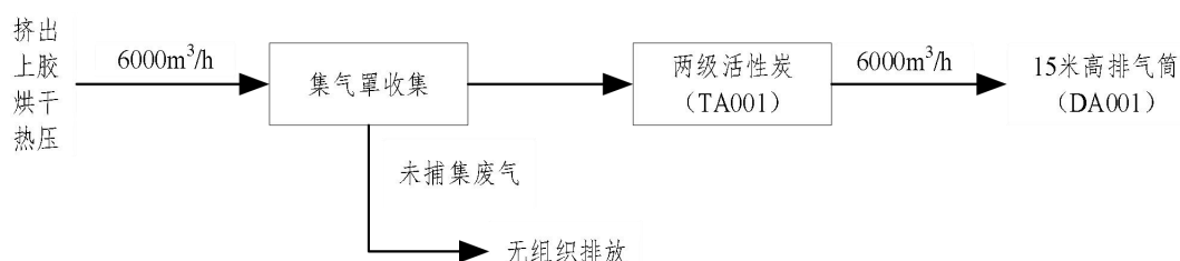
图 4-1 企业废气处理工艺图
