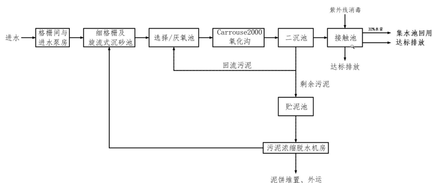
图 4-2 污水处理厂工艺图
